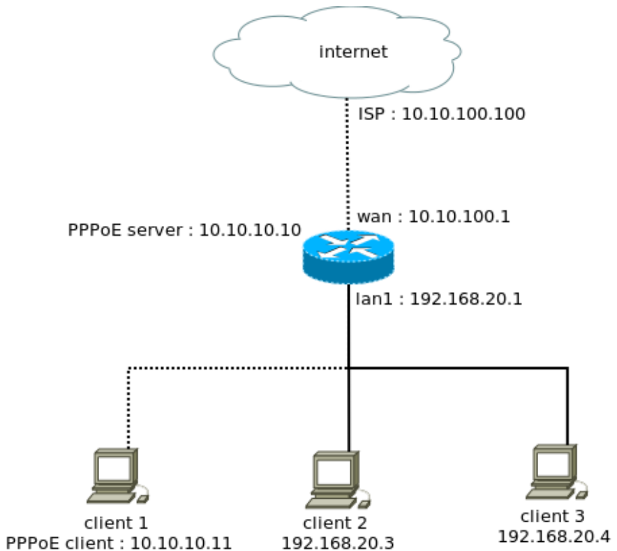
Gambar 8.18 Jaringan PPPoE
