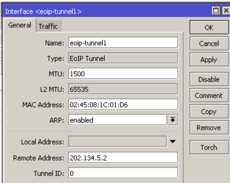
Gambar 8.5 EoIP Interface kota B
