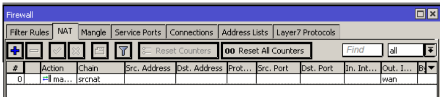
Gambar 2.22 Hasil konfigurasi NAT
