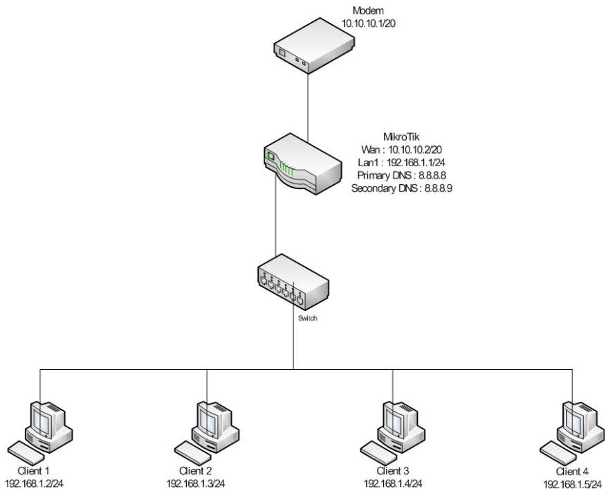
Gambar 2.19 Topologi Mikrotik Internet
