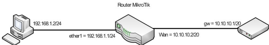
Gambar 2.13 Topologi jaringan
