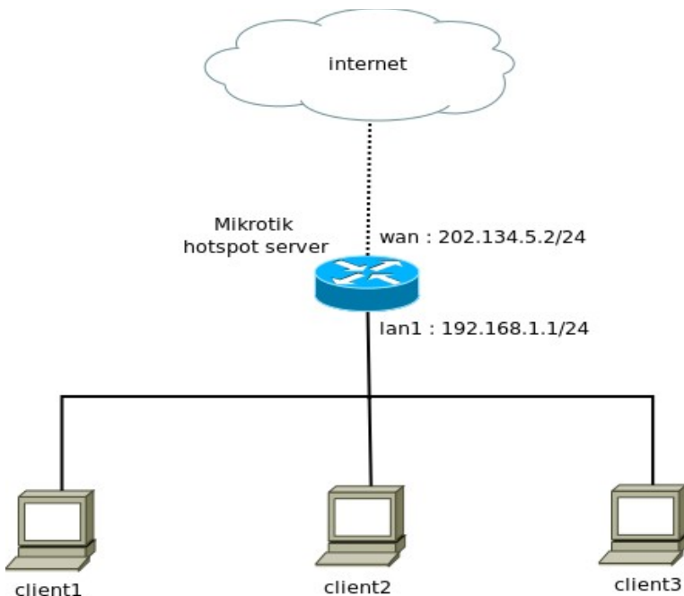
Gambar 6.1 Hotspot Mikrotik
